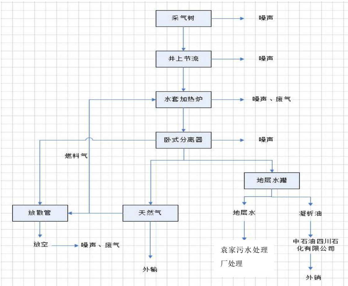
图 2.4-1 天然气开采工艺流程及产污节点图
