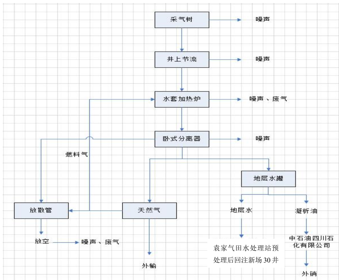
图 2.3-1 天然气开采工艺流程及产污节点图
